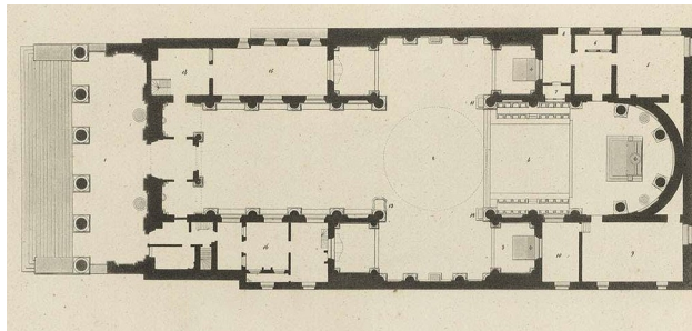
Plan de l'église en 1827 de Pierre-Jacques Goetghebuer les quatre chapelles sont encore apparentes parvis à gauche (ouest)
